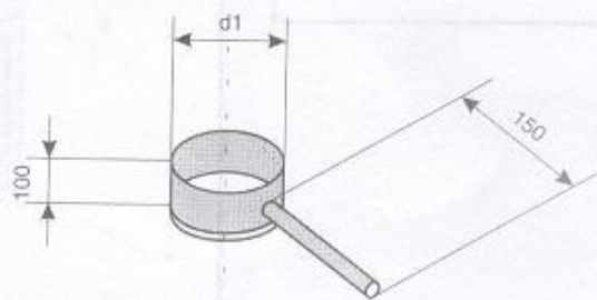
Z odpływem bocznym
