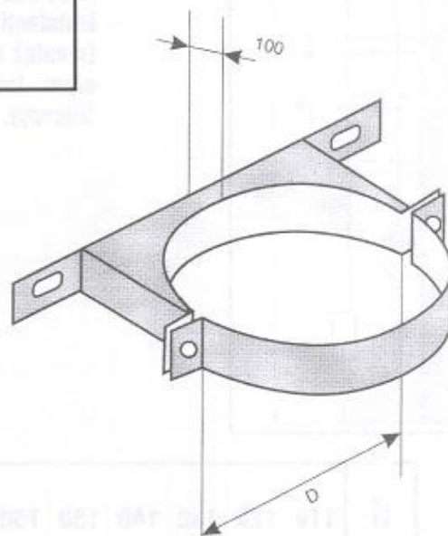
UMD Uchwyt mocujący kominą
