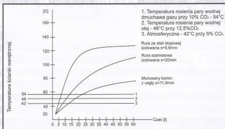
Rozkład temperatur wewnątrz przewodów odprowadzających gazy spalinowe w różnych systemach kominowych w fazie nagrzewania.
