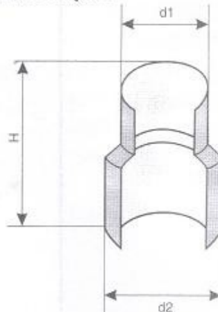
RR Redukcja rozciągana
