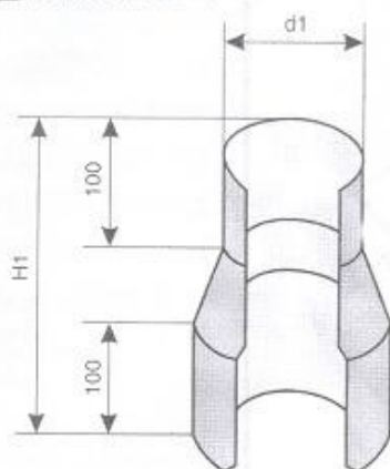
RS Redukcja stożkowa
